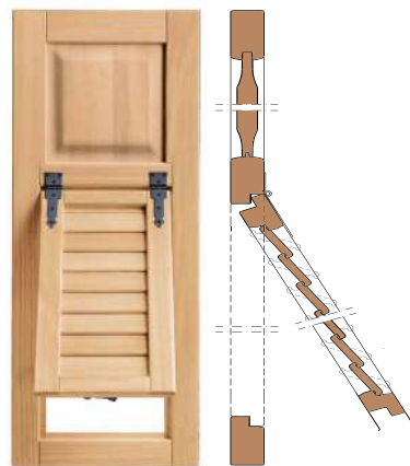
T07 Mit Aussteller, nicht bewegliche Lamellen
